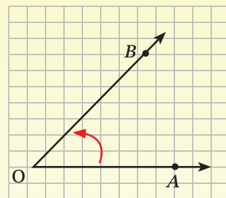
(A\hat{O}B)
