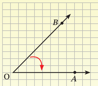
(B\hat{O}A)
