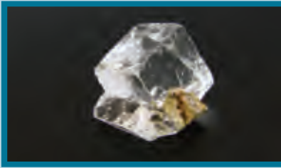
شكل 38 معدن الكالسيت Calcite
