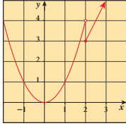
شكل (7) يمثل بيان الدالة في مثال (6)
