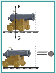
(شكل 104) تساوي القوة التي تؤثر في القذيفة، لدفعها إلى الأمام في المقدار، وتعاكس في الاتجاه مع قوة ارتداد المدفع إلى الخلف.
