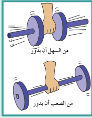
(شكل 64) يعتمد القصور الذاتي الدوراني على بعد الكتلة محور الدوران.
