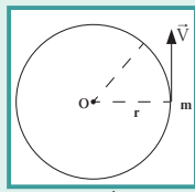
(شكل 82) كتلة نقطية تدور بسرعة مماسية v حول محور في مسار دائري.
