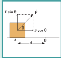
(شكل 4) تحليل القوة بمتجهين المتجهات لقوة F تصنع زاوية \theta مع اتجاه الحركة.
