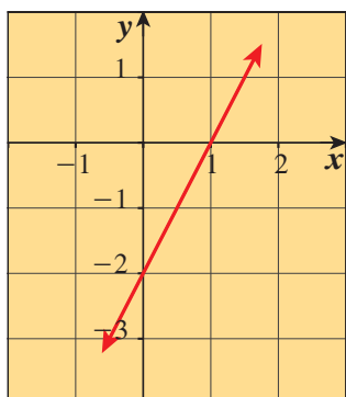
شكل (1) بيان الدالة f'
