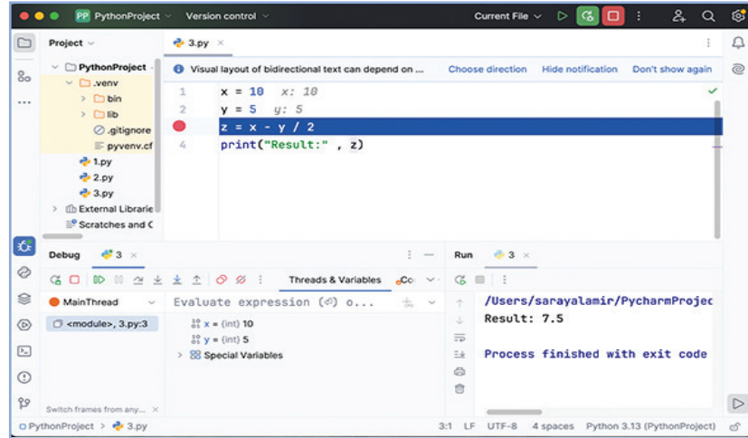
شكل (3-7) يوضح بعض أدوات تتبع الأخطاء في PyCharm.
