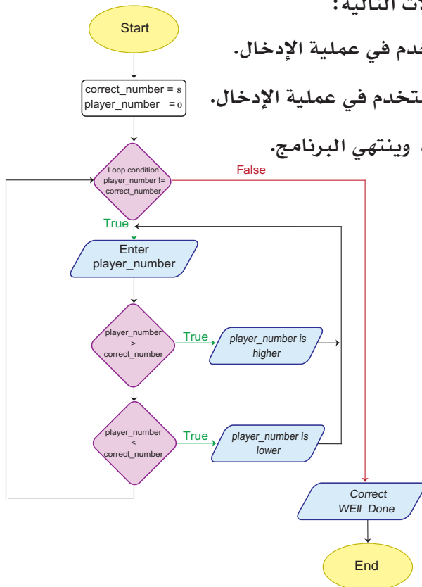
شكل (6-7) خريطة تدفق برنامج تخمين عدد صحيح.
