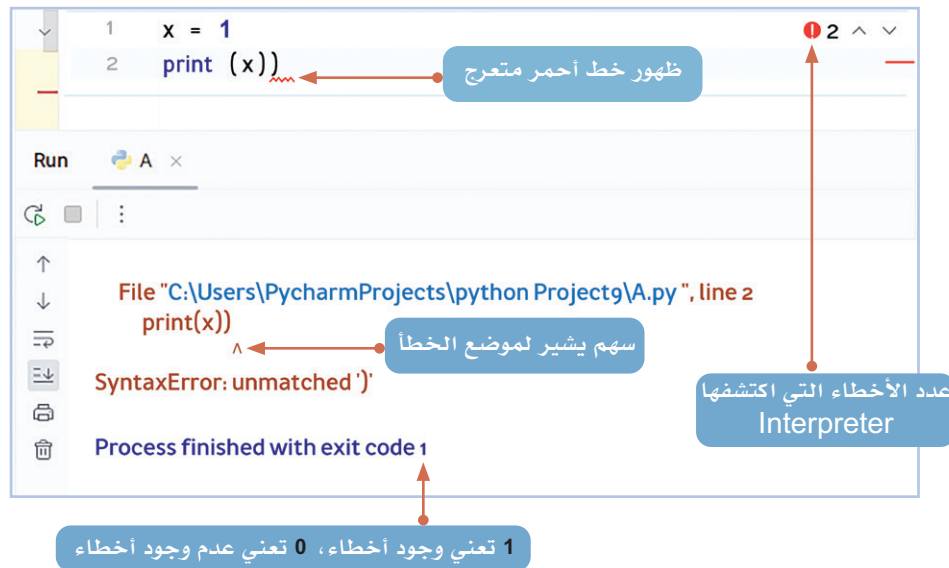
شكل (2-7) يوضح اكتشاف خطأ في بناء الجملة Syntax Error، وتحديد موضعه في بيئة البرمجة.
