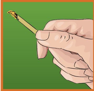
(أ) عند إشعالها في الهواء
