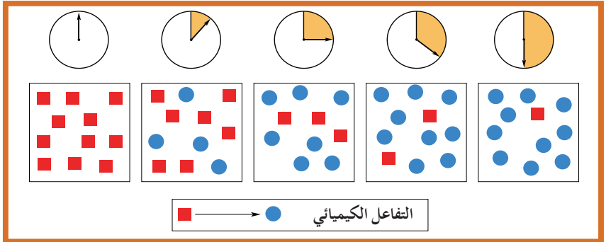
شكل (33) مع مرور الوقت، تتناقص كمية المتفاعلات (المرتبات الحمراء) وتزداد كمية النواتج (الدوائر الزرقاء).
