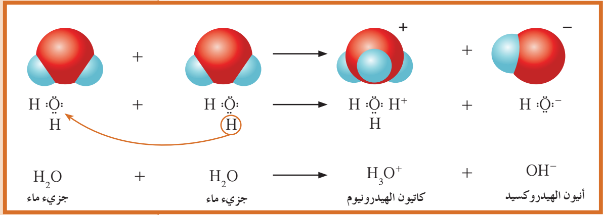
شكل (59) تفاعل التأين الذاتي للماء
