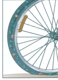
ضغط منخفض: جسيمات غاز أقل داخل الإطار
