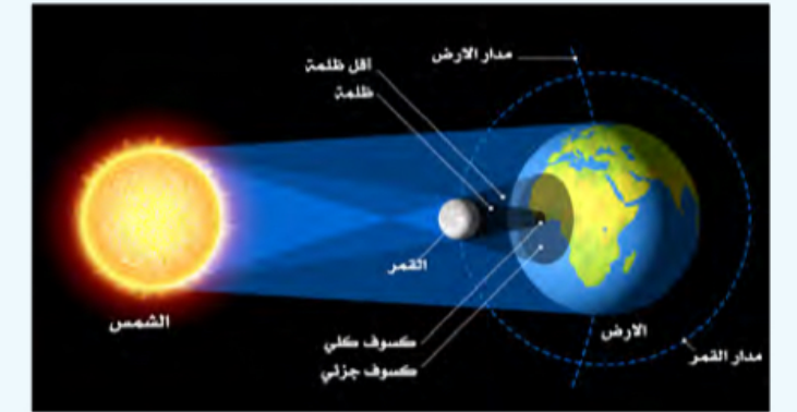
الكُسُوفُ
