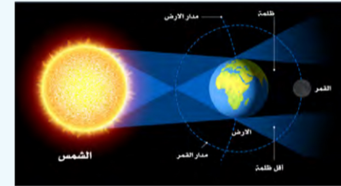
الخُسُوفُ
