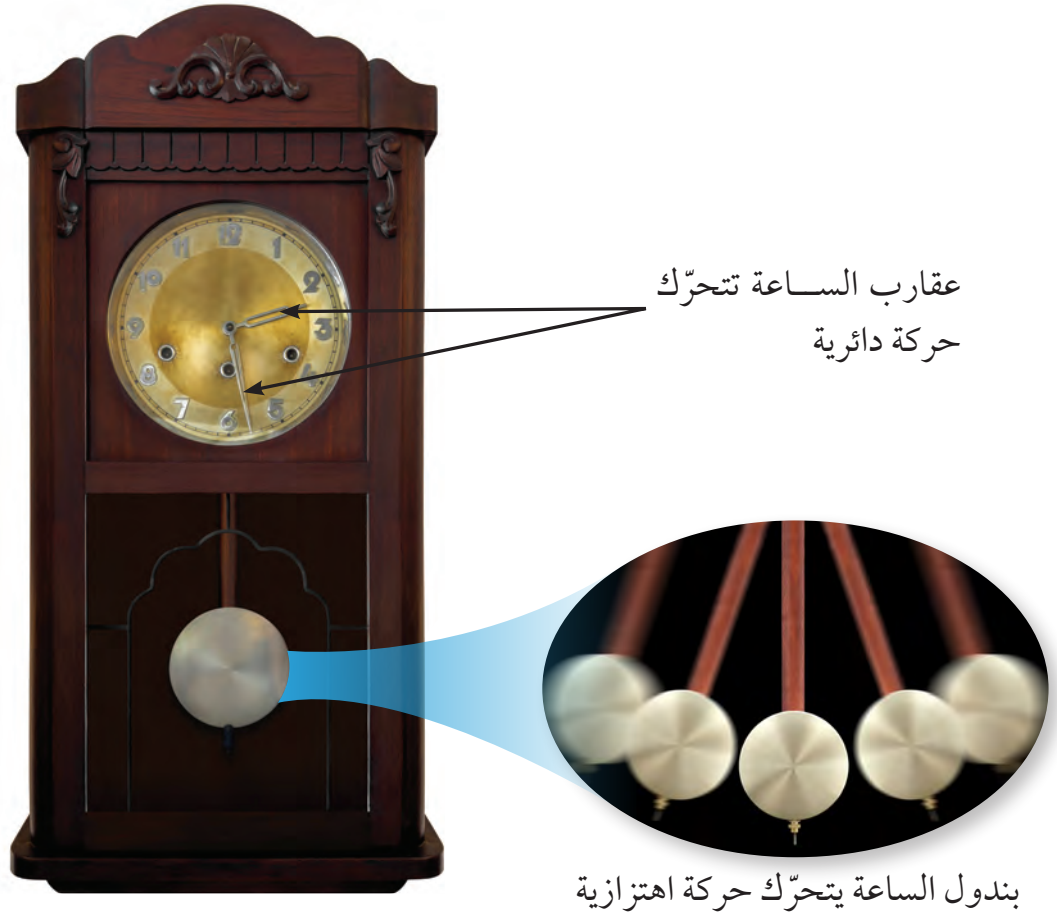
الشكل (١٢) الحركة الدورية
