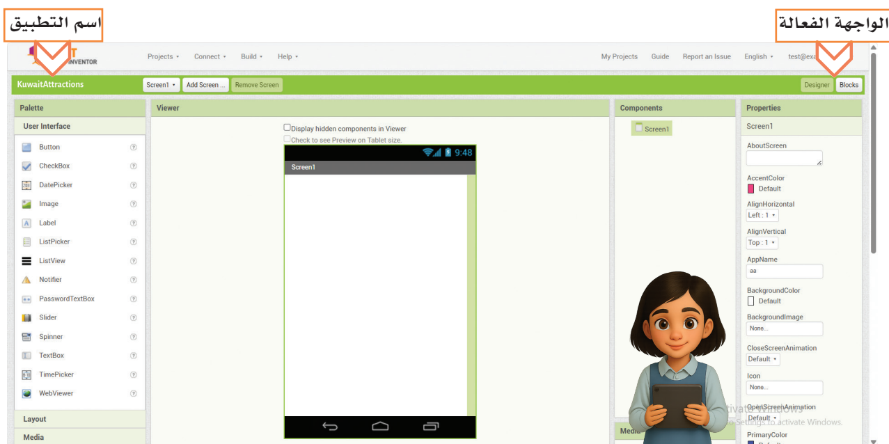
شكل رقم (9): الواجهة بعد انشاء مشروع جديد
