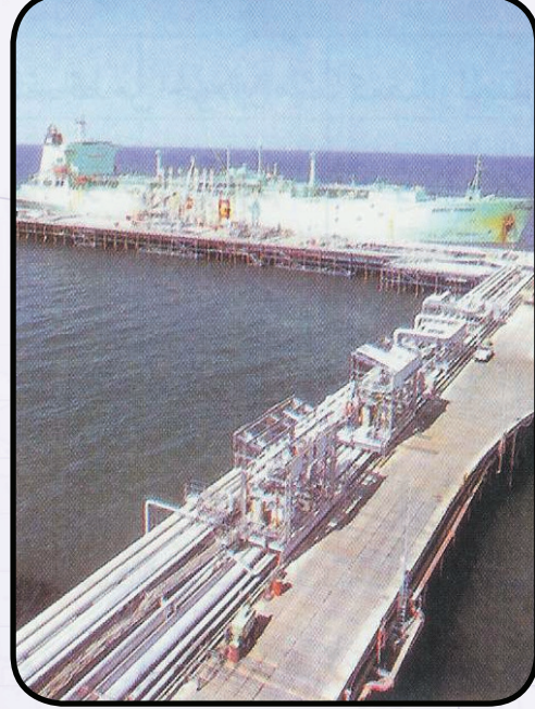
شكل (٧-٥) محطة تحميل النفط في الرصيف الجنوبي
