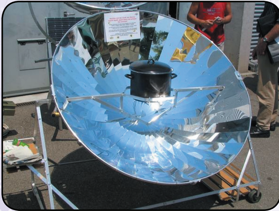
شكل (٣-٢) - الطباخ الشمسي
